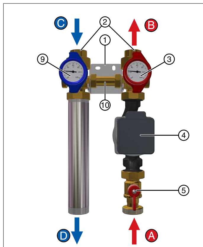
Fig. 7: Structure du module HK25-KH
