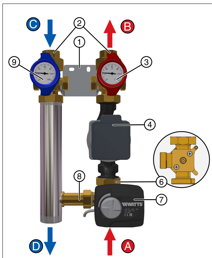
Fig. 6: Structure des modules HKM25 et HKM32
