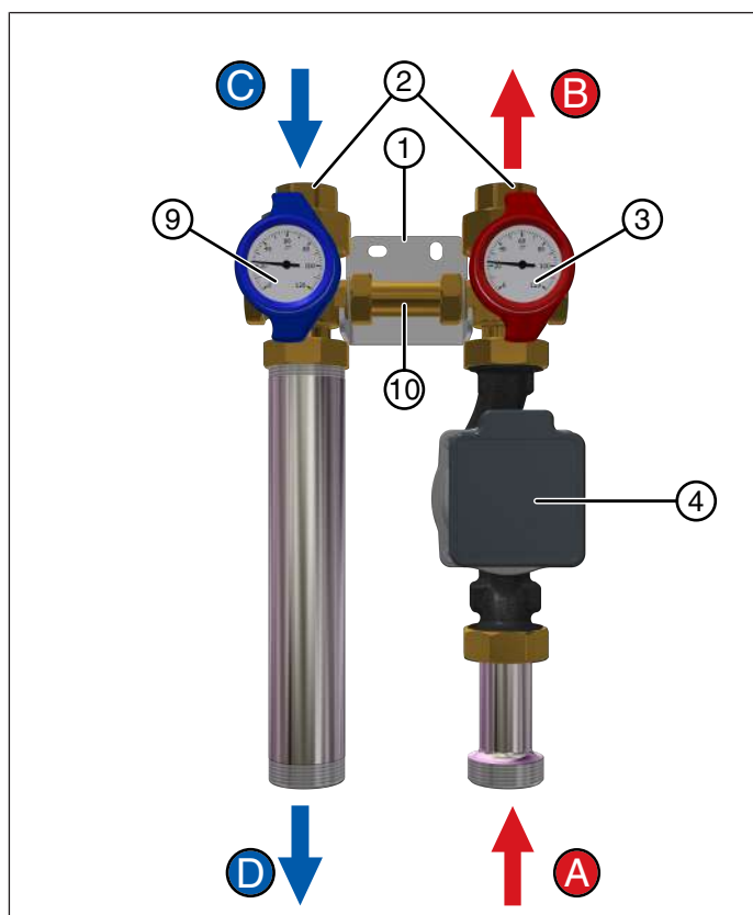
Fig. 5: Structure des modules HK25 et HK32
